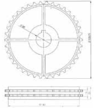
12.7 HASIRBAND DIŞLI Z.38 Göbek: Ø25mm Ø30mm 40.40 kare
