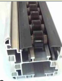
106X120 Alüminyum Sigma Profil Montaj Hattı için 106X120 Assembly Line Aluminium Profile
