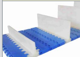
25,4 Hasır Bant için Götürücü Cleats for Modular Conveyor Belts
