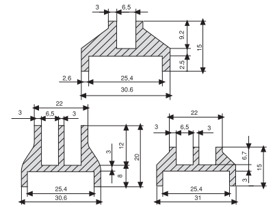
Açılır Çerçeve Profilleri Runner Profiles
