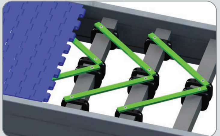
12,7 Hasır Bant Modular Conveyor Belts
