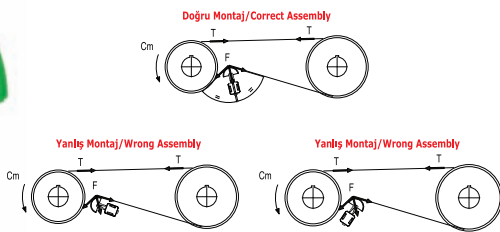
Zincir Gergi Aparatı Chain Tensioner
