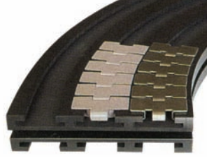
Alpolen 1000, 90° (880 Tab 881 Tab Dönüşlü Bantlar İçin) Curves Track for 880 TAB-881 TAB chains
