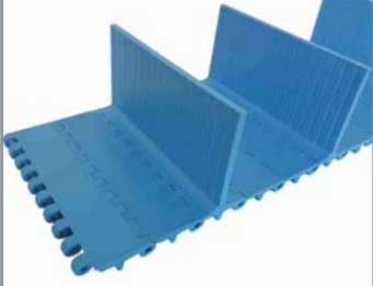
50,8 Götürücülü Kolay Temizlenebilir Bant 50,8 Easy to Clean Conveyor Belts
