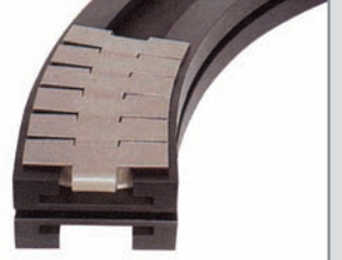
Alpolen 1000, 90° Dönüş Yatakları (882 Tab Dönüşlü Ağır Tip Bantlar İçin) Curves Track for 882 TAB chains/heavy duty)
