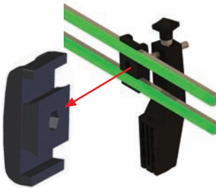
Balık Sırtı Profil İki Mengene Double Clamp with Rod
