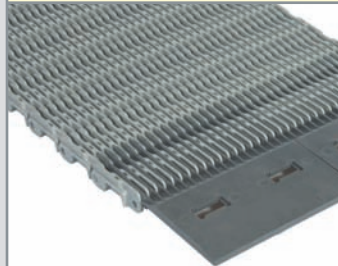
50,8 Kaburgalı Kanallı Hasır Bant (Ağır Tip) Raised Rip Modular Conveyor Belts
